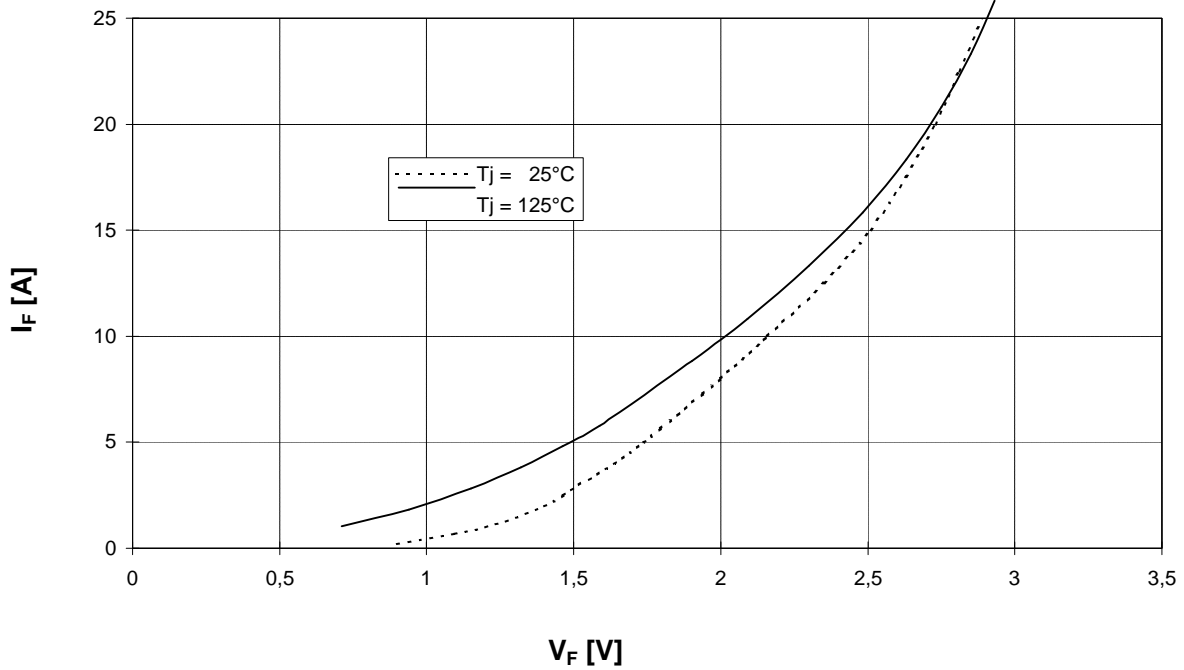
Durchlaßkennlinie der Brems-Chopper-Diode (typisch) Forward characteristic of brake-chopper-FWD (typical)
